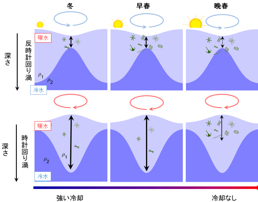
図 2：反時計回り（上）と時計回り（下）の渦での植物プランクトンの増加メカニズムの違い 反時計回りの渦では太陽光が少し強くなることで植物プランクトンが増加を始めるが、時計回りの渦では表面の海水が混ざりにくくなって初めて植物プランクトンの増加が始まる（矢印は混合の深さと強さを示す）
