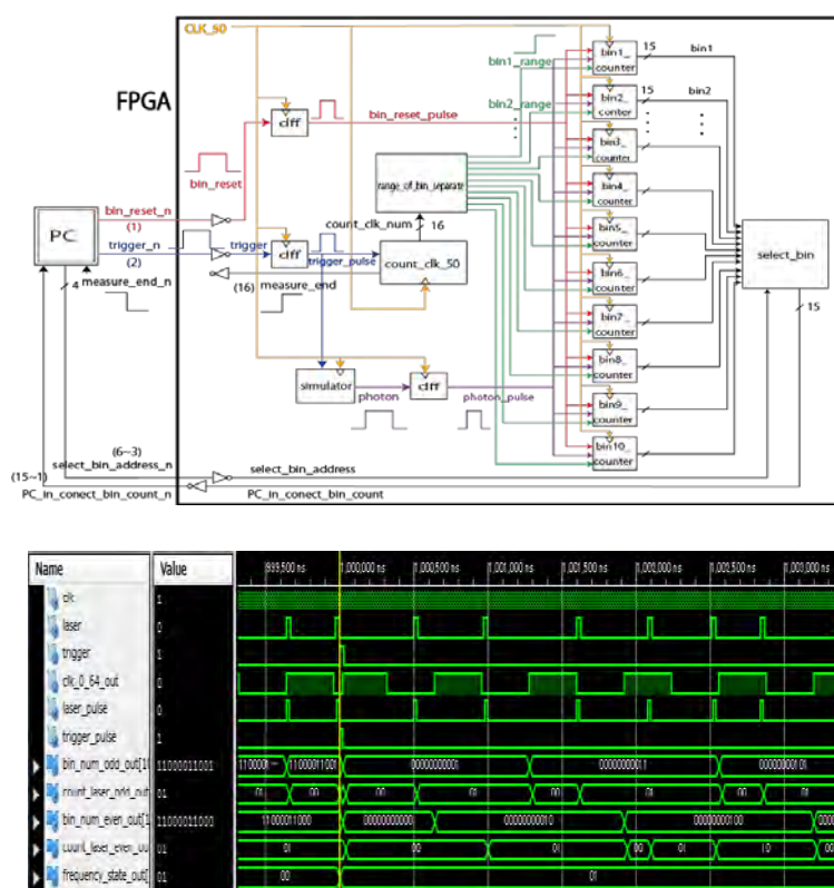
図1 (上) FPGA を用いたカウンタの構成図 (下) カウンタシミュレーションのテスト画面
