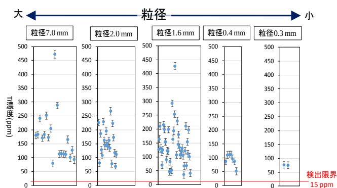
図 2 粒径 (0.3 mm~7.0 mm) と Ti 濃度の関係
