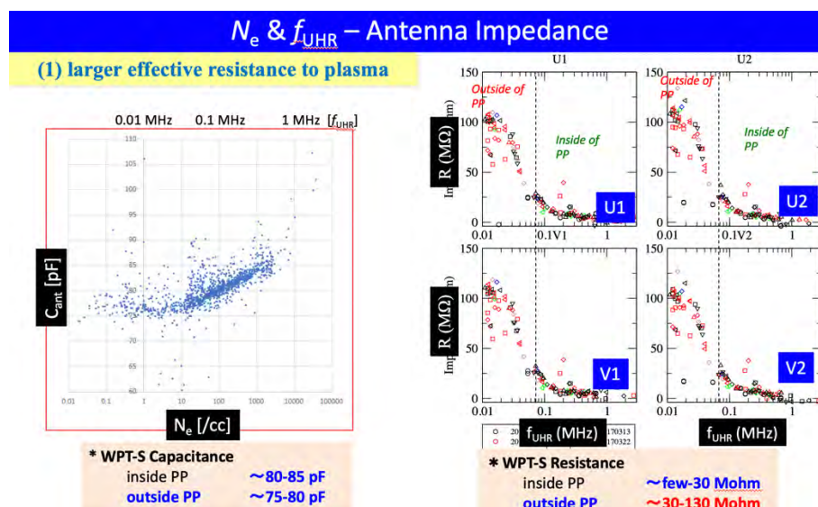
図 1: 暫定的な Probe impedance 評価結果。左:Capacity、右:Resistance
