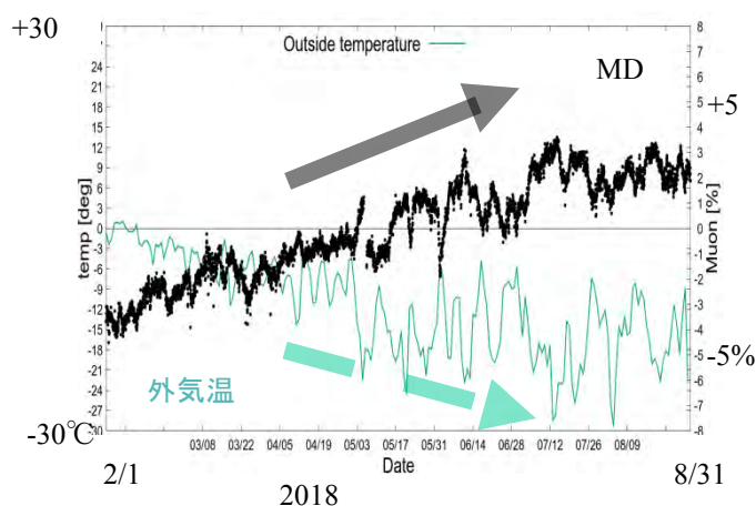
図1 観測されたミュオンの負気温効果
