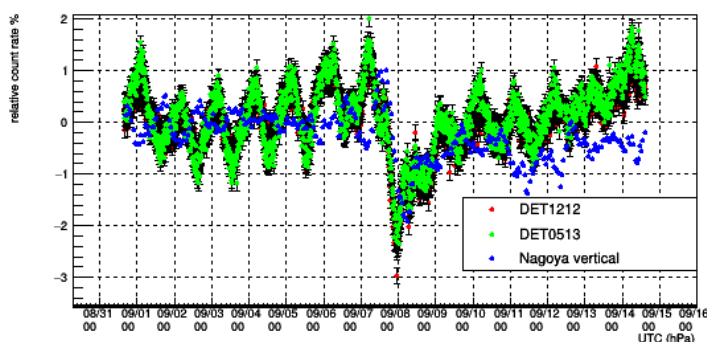
図 3: TA 実験検出器と名古屋大学ミュオン計の比較
