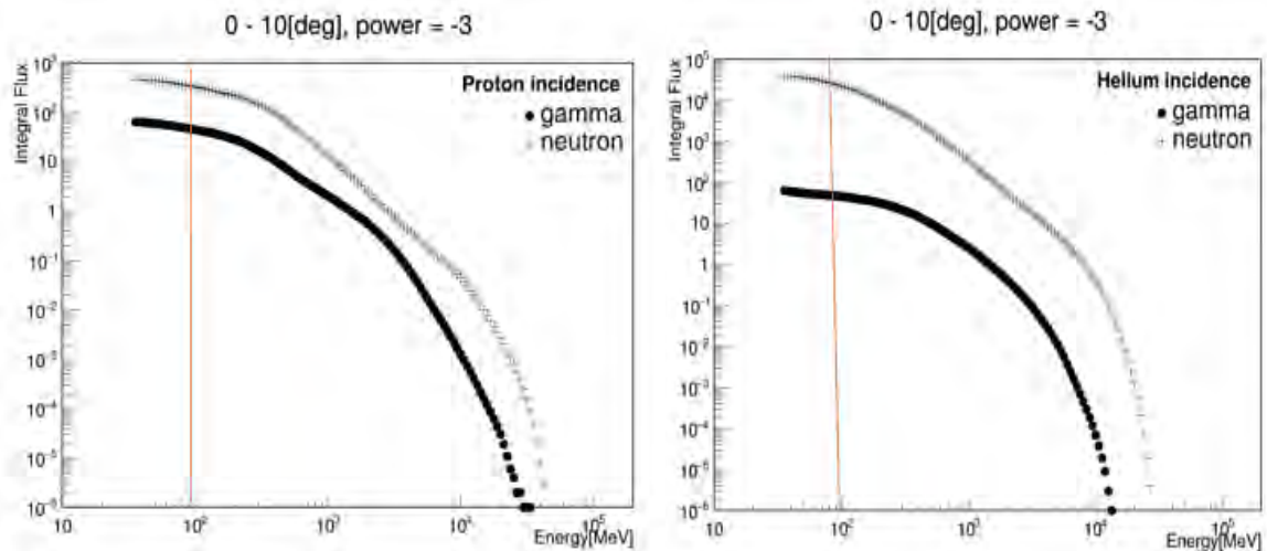
図 6 陽子(左) と ヘリウムイオン(右)が太陽大気と衝突して作り出すガンマ線 (●) と中性子 (+) の積分エネルギースペクトル。 100MeV に引かれた縦線は FERMI-LAT の観測閾値に対応している。SEDA-FIB は 35MeV 以上の中性子を検出できるが、ここでは FERMI-LAT の閾値と合わせるために >100MeV 以上の中性子を選択している。ヘリウムイオンが太陽大気に衝突した時は n/\gamma 比に約 1000 倍の値が予想される。これは加速された原子核が衝突により陽子と中性子に破碎され、その中性子が太陽から地球にやってくるためである。加速イオンのべきは 3 \text{乗}(E_{\text{ion}}^{-3}) を仮定し、観測点は太陽大気の厚みは 10\text{g/cm}^2 の地点としている。現実には様々な化学組成でもって衝突するのでこのグラフのように 1000 倍にはならないだろう。
