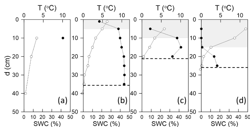
図1：SPおよびEGにおける(a)連続測定、(b,c,d)手動測定による活動層内の温度T(○)と土壌体積含水率SWC(●)の鉛直プロファイル。網掛けは有機物堆積層、破線は融解深度を示す(2018年6月22–23日EGサイト)。
