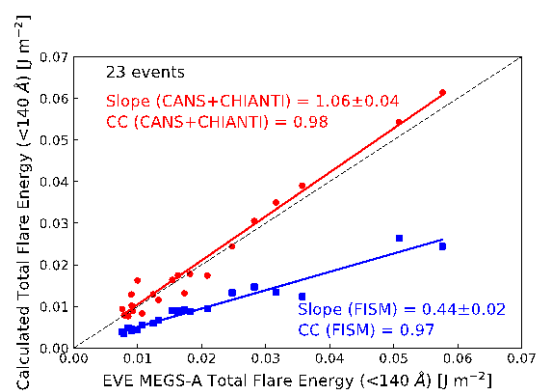
図2 フレアにおけるEUV放射エネルギー(<140Å)の数値計算モデル(CANS+CHIANTI, FISM)の値と観測値(SDO/EVE)との比較。
