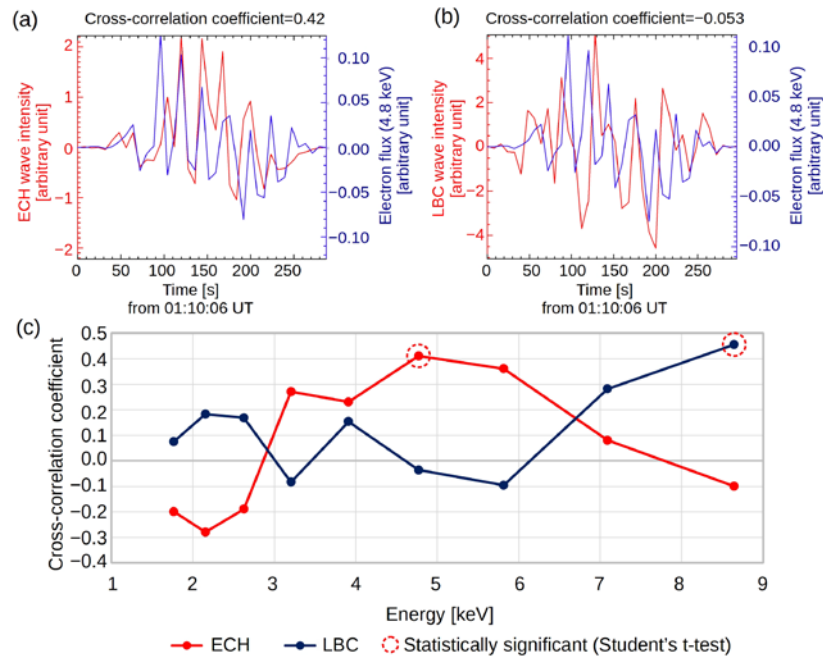
図 1 (a) ECH 波強度 (赤線) と 4.8 keV のロスコーン内の電子フラックス (青線)。 (b) コーラス波強度 (赤線) と 4.8 keV のロスコーン内の電子フラックス (青線)。 (c) ロスコーン内の電子フラックスと ECH 波との相互相関係数 (赤線) およびロスコーン内の電子フラックスとコーラス波との相互相関係数 (青線)。
