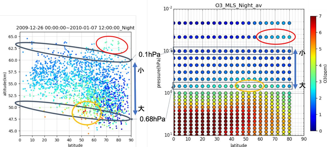
(図1) 左は本シミュレーション、右はAura/MLSで観測されたオゾン混合比の緯度高度断面図。両者の分布はよく似た傾向を示すが、シミュレーションのほう観測よりも全般的に値が大きい。
