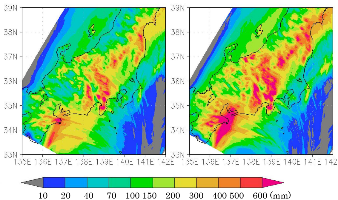
図 2 : 令和元年台風 19 号での再現された積算降水量 (左) と将来気候を仮定した実験での降水量 (右)
