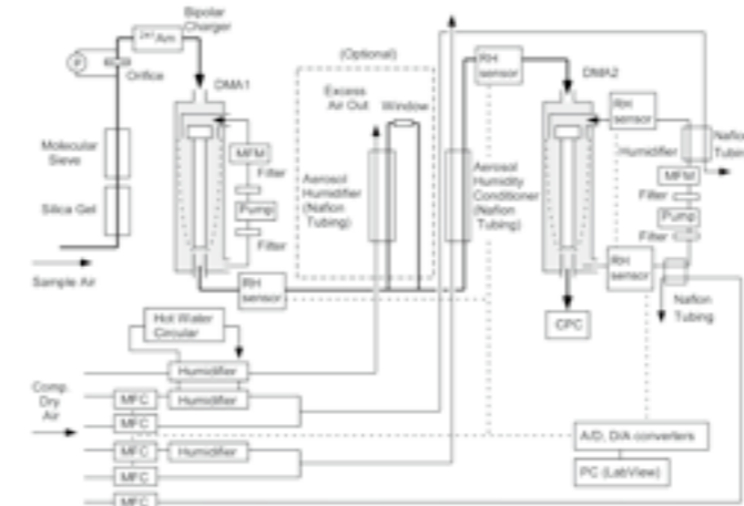
エアロゾル粒子の吸湿成長度を測定するために使用する吸湿特性測定用タンデムDMA (HTDMA) の構成
