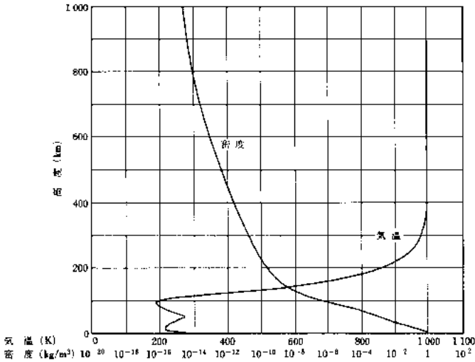
気温、密度の高度分布
