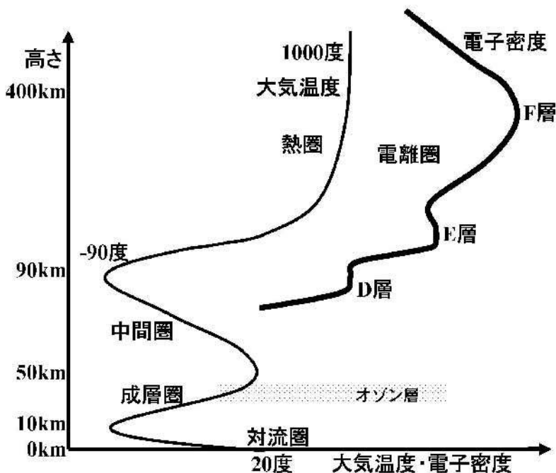
大気の温度構造とそれぞれの高さの名前。
