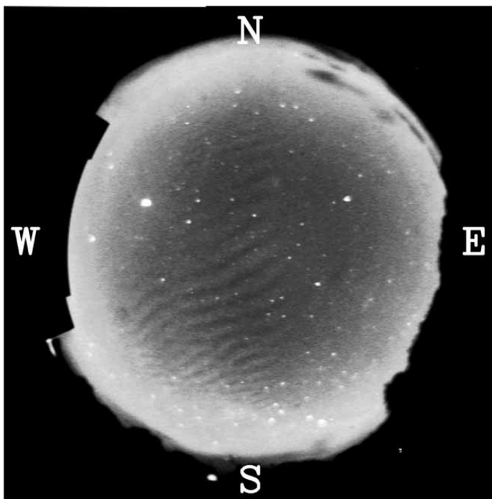
大気光を通して観測した中間圏の大気重力波の画像。特に左下の部分に南西から北東方向に波面を持つ大気重力波が見える。白い点は星。
