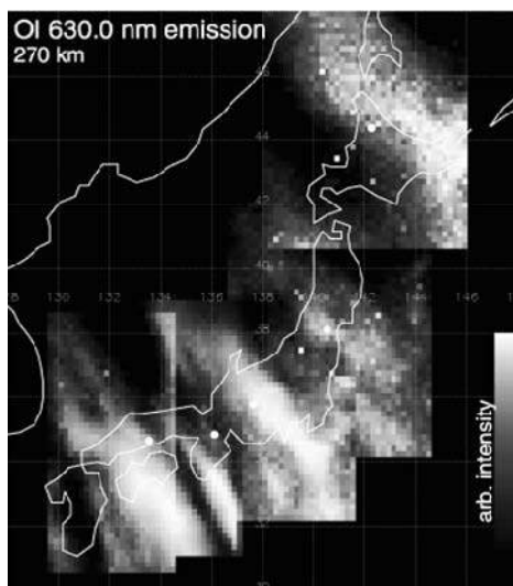
日本列島を南西に向けて横切る電離圏のしましま構造 （地上5カ所で同時に撮影された大気光の合成画像）。
