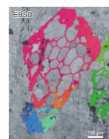
ハニカム構造を示すざくろ石のEBSDマップ(三波川変成帯 石英片岩)。
