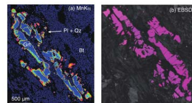
セグメント化したざくろ石の (a) EPMA MnK・マップと(b) EBSD マップ(ミャンマー・Mogok グラニュライト)。鉱物の略号: Bt: biotite, Gtr: garnet, Pl: plagioclase, Qz: quartz.
