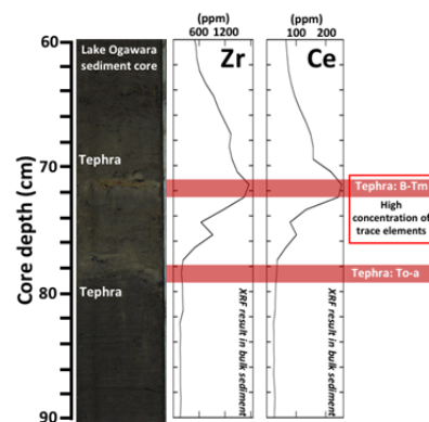
小川原湖堆積物の Zr、Ce 鉛直分布図と堆積物写真。
