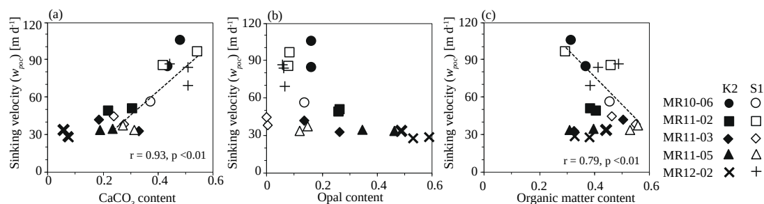
亜熱帯域 S1 (30°N, 145°E) と亜寒帯域 K2 (47°N, 160°E) におけるトラップ粒子の平均沈降速度と(左) \text{CaCO}_3 、(中) オパール、(右) 有機物含有率の関係。
