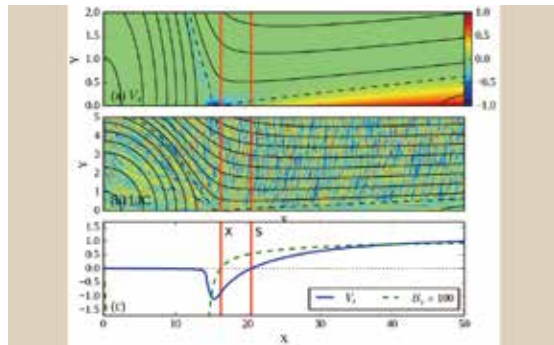
非定常ベッチェック型磁気リコネクションのシミュレーション (本文 P51 参照)。
