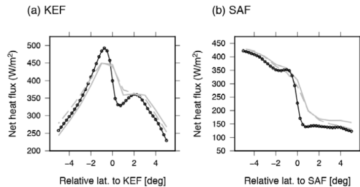
北太平洋の主要な海洋前線に伴う海面フラックス変動：海面水温で規定される海洋前線を中心とした 1 月の気候学的月平均より。黒潮主流前線（左）、亜寒帯前線（右）、黒色：本研究（J-OFURO3）、灰色：これまでのデータセット（J-OFURO2、OAFlux）。
