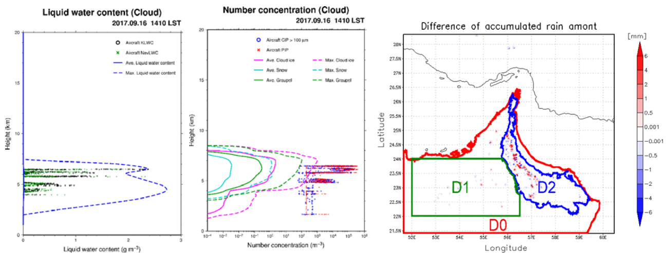
図1: 観測(点線)とモデル(破線)から得られた雲水量濃度(左図)と降雪粒子数濃度(中央図)の比較。雲核数濃度を標準値500個 \text{cm}^{-3} から倍増させた場合の地上降水量の増減分布(右図)。
