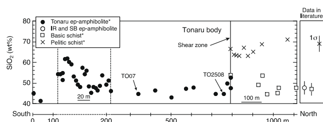
国領川ルートに沿う全岩 SiO 2 量の変化。
