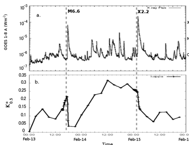
2011 年 2 月 13 日から 15 日までの (a) GOES X 線流束と (b) \kappa^* の時間変化。2 つの破線は活動領域 NOAA 11158 で発生した大型フレアの時間を示す。
