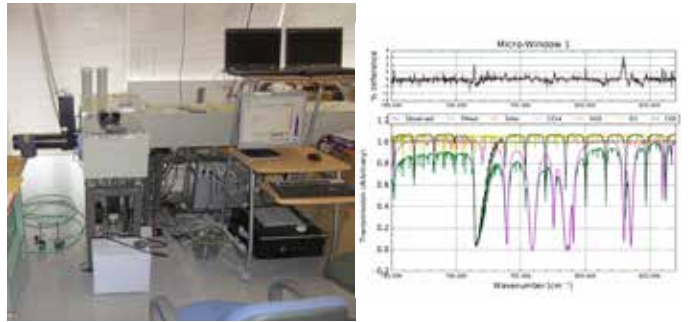
陸別観測所で稼働している高分解能 FTIR (国立環境研究所が保有) (左) と観測されたオゾン、水蒸気、二酸化炭素及び四塩化炭素の吸収スペクトル (右)
