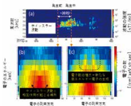
あらせ衛星が観測したプラズマの波（上）と、電子の分布（下）。上の段のホイッスラー波動が発生すると、電子の分布が下左から下右へと変化し、電子が加速していることが発見されました。（Kurita, Miyoshi et al., 2018 を改訂）
