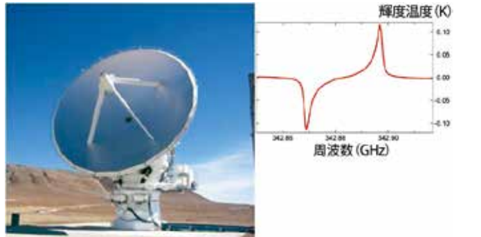
ASTE 望遠鏡 (左) で木星の硫化炭素 (CS 2 ) を観測した場合のシミュレーションスペクトル (右)
