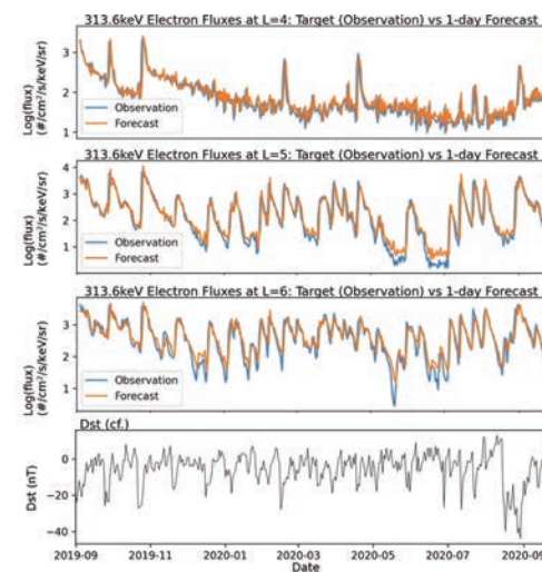
左：「あらせ」衛星の観測データの機械学習に用いたニューラルネットワーク 下：機械学習によって予測した放射線帯電子の変動と実際の観測結果との比較
