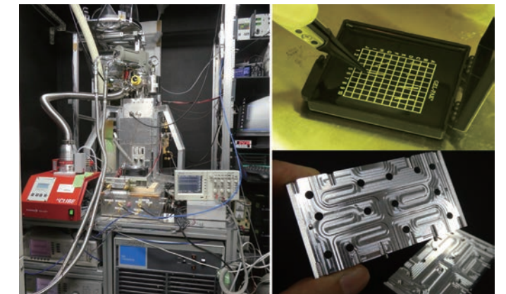
ノルウェーに設置したミリ波ラジオメータの外観 (左)。大学院生と共に設計開発を行った超伝導検出素子 (右上) および導波管型周波数分配器 (右下)
