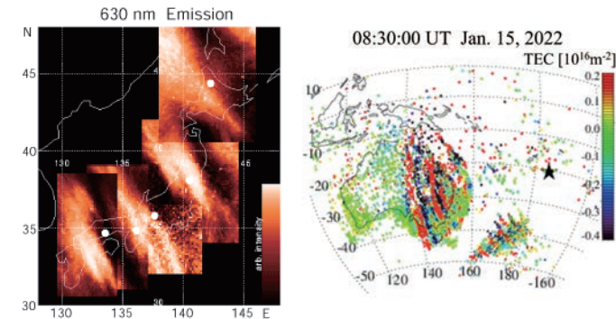
(左) 日本列島上空を北東から南西へ伝搬する MSTID の大気光観測 (右) トンガの火山噴火後に GPS で観測された電離圏変動
