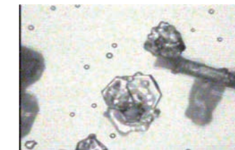
(上) 2013年6月15日にパラオ共和国で放球された雲粒子ゾンデ HYVIS により取得された雲粒子と固体降水粒子の画像
