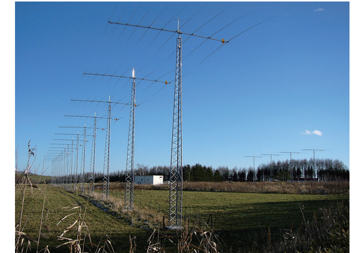
北海道-陸別短波レーダーの巨大なアンテナ群
