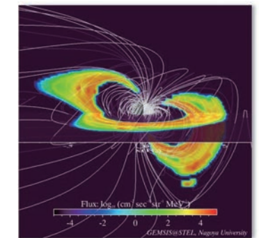
ジオスペース放射線帯電子変動のシミュレーション
