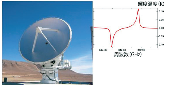
ASTE 望遠鏡 (左) で木星の硫化炭素 (CS) を観測した場合のシミュレーションスペクトル (右)
