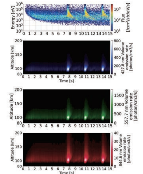
オーロラを起こす電子および異なる波長でのオーロラ発光の数値シミュレーション
