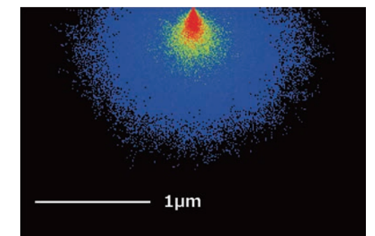
モナザイト中のトリウム M 線の発生領域 (シミュレーション)
