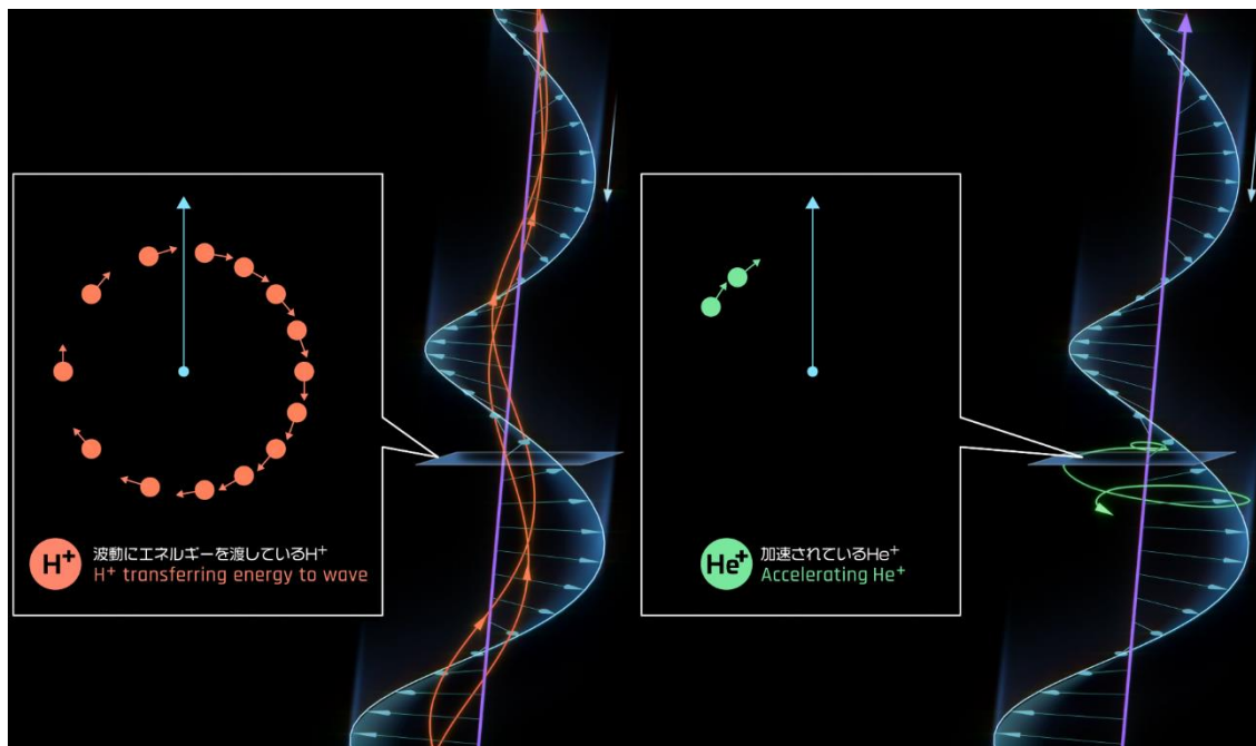
図 2: 観測されたジャイロ非等方の模式図 (コピーライト: 東京大学)
