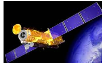
太陽観測衛星「ひので」 （2006年打ち上げ） ©国立天文台 / JAXA
