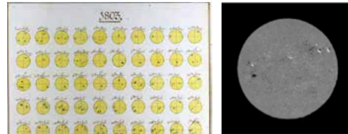
左：オーストリアの図書館に収蔵されている200年前の手書きの黒点スケッチ 上：機械学習を用いて手書きの黒点スケッチから再現した200年前の太陽表面磁場
