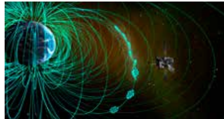
ジオスペース探査あらせ衛星（2016年打ち上げ） ©ERG サイエンスチーム
