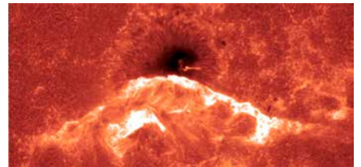
「ひので」衛星が観測した太陽黒点およびフレア ©国立天文台 / JAXA
