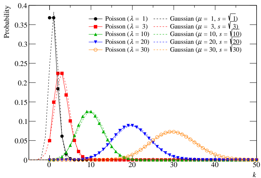
図 10.3 様々な平均値を持つポアソン分布と正規分布の比較
